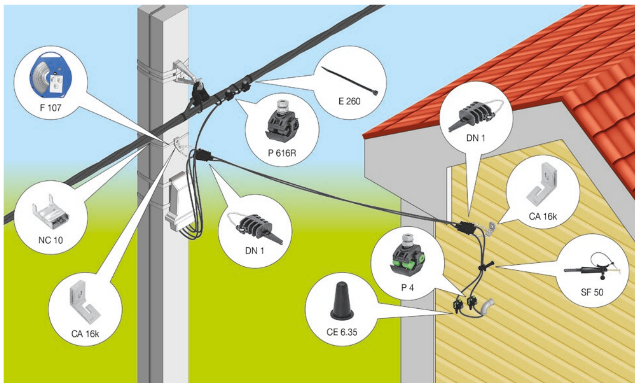
Представленная схема соответствует типовому проектному решению ОАО «НИИЦ МРСК»
