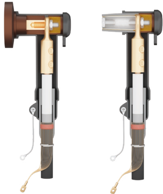
Визуализация подбора адаптеров
