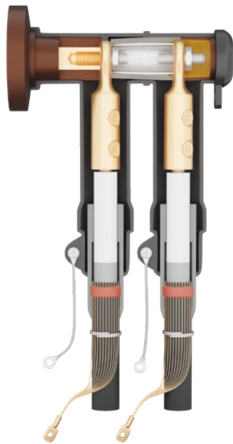
Двойное подключение HICS-5851+ HICS-CC-5851
