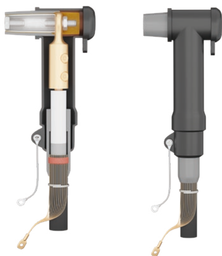
Второй адаптер для двойного подключения
