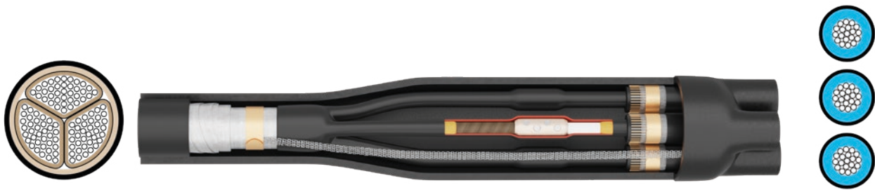
3-х жильный кабель с бумажной изоляцией в отдельных оболочках и одножильный кабель с пластмассовой изоляцией
