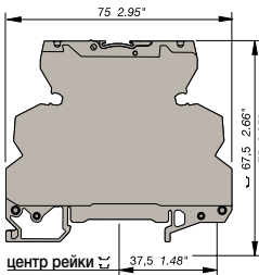
Модуль с пружинным
