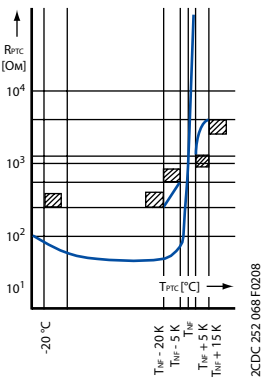
Характеристики датчиков температуры
