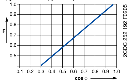
Поправочный коэффициент F для индуктивной нагрузки переменного тока
