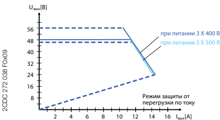
CP-T 48/10.0 режим защиты от перегрузки по току
