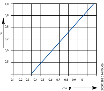
Кривая снижения ном. параметров
