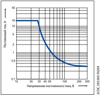
CR-P с 1 переключающим контактом
