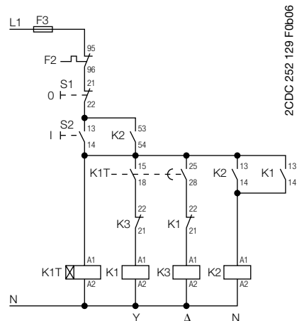
Схема управления
