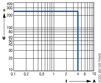
Кривая снижения ном. параметров
