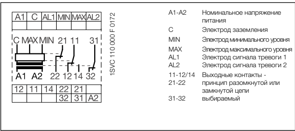
Схема подключения CM-ENN UP/DOWN
