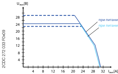
CP-T 24/20.0 U/I кривая
