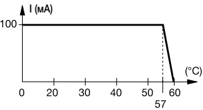
D 2,5/5-OBOC-0100 5 В пост. тока / 24 В пост. тока
