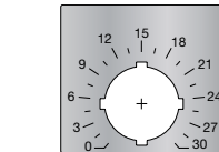
Шильдик со шкалой 0-30 48,5 x 44,5 мм
