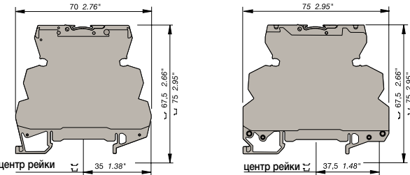
Модуль с винтовым зажимом
