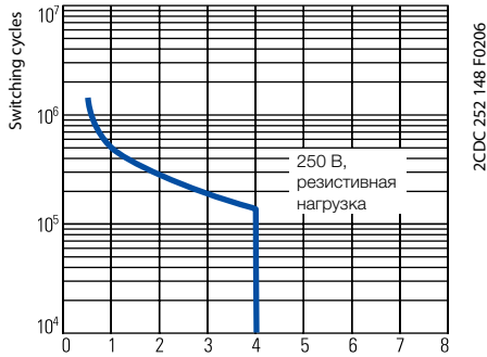
Срок службы контактов
