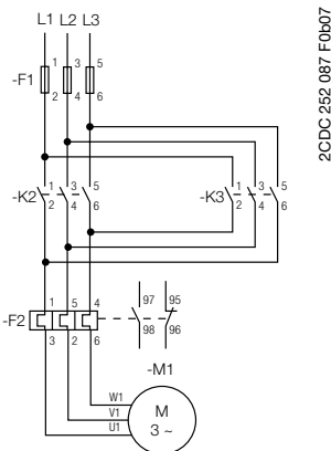
Схема электропитания
