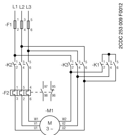
Схема питания
