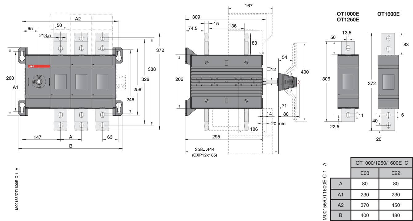
OT1000 ... 1600E03C (в сборе с ручкой ОНВ200J12PE011 и переходником ОХР12х185)
