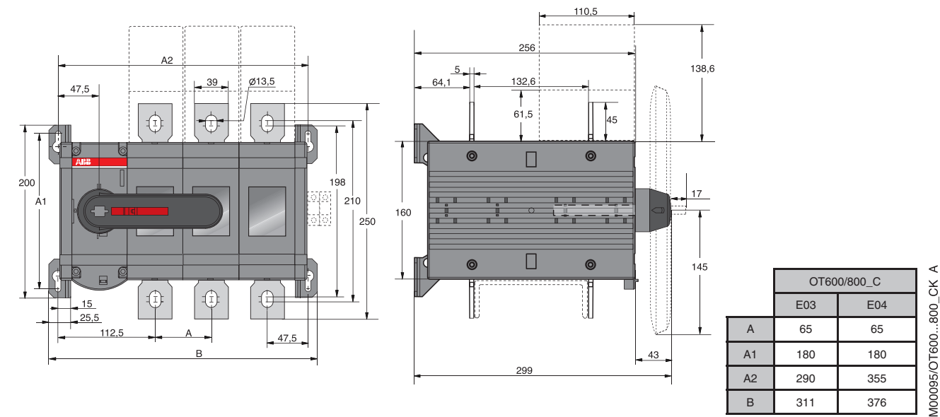
OT630E03/04C ... 800E03/04C (в сборе с ручкой прямого монтажа OTV800ECK)
